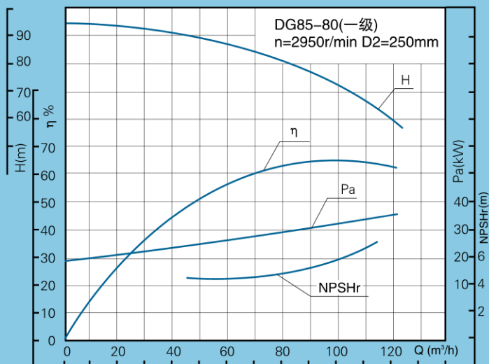
DG85-80次高压泵性能曲线表
