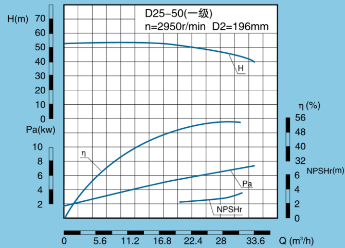
D、DG、DF、DY、DM25-50 性能表
