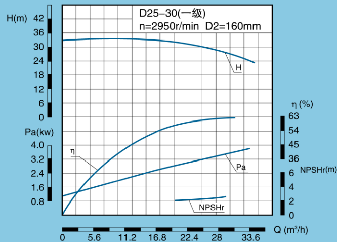
D、DG、DF、DY、DM25-30 性能表
