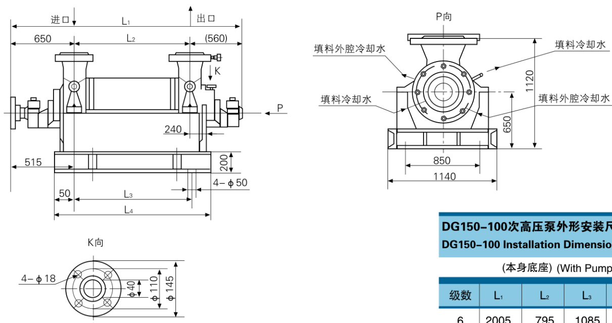
DG150-100型次高压泵外形安装图
