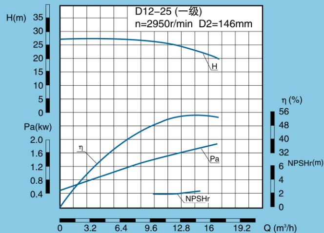
D、DG、DF、DY、DM12-25 性能表
