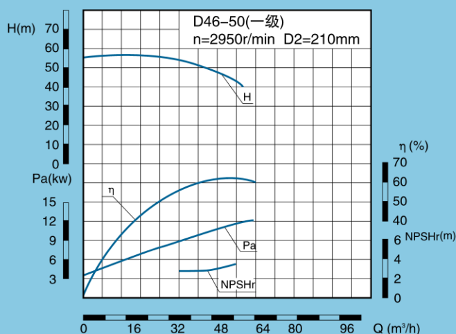
D、DG、DF、DY、DM46-50 性能表
