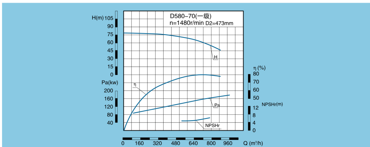
D、DG、DF、DY、DM580-70性能表 D、DG、DF、DY、DM580-70 Performance Data
