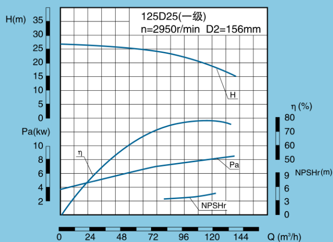
125D、DG、DF、DY、DM25 性能表
