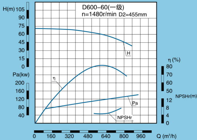
D、DG、DF、DY、DM600-60性能表 D、DG、DF、DY、DM600-60 Performance Data
