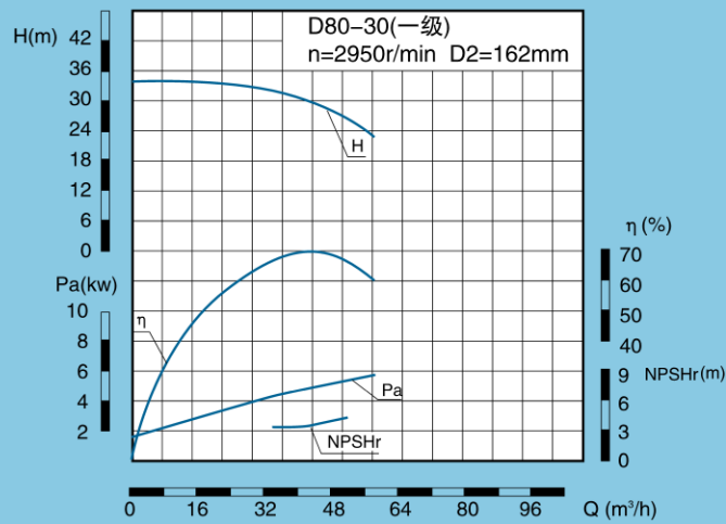
D、DG、DF、DY、DM80-30 性能表
