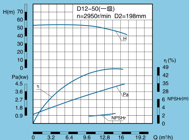
D、DG、DF、DY、DM12-50 性能表
