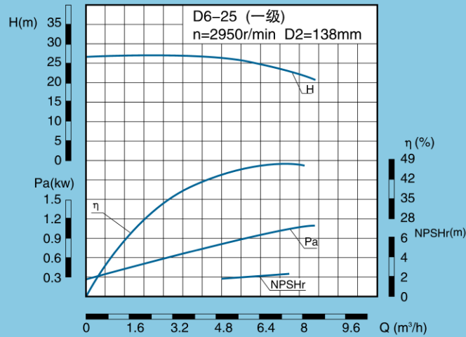
D、DG、DF、DY、DM6-25 性能表
