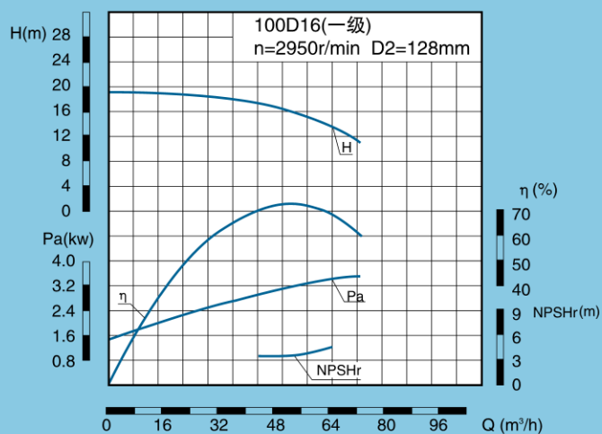
100D、DG、DF、DY、DM16 性能曲线
