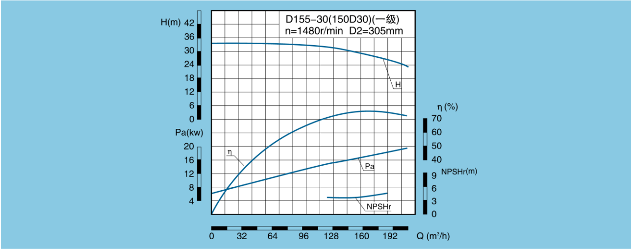
D、DG、DF、DY、DM155-30(150D30) 性能曲线 D、DG、DF、DY、DM155-30(150D30) Performance Curve
