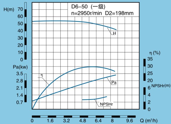
D、DG、DF、DY、DM6-50 性能表
