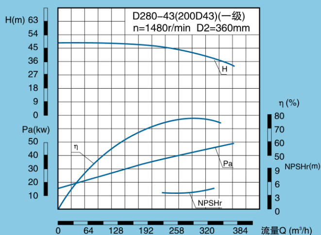
D、DG、DF、DY、DM280-43(200D43) 性能表
