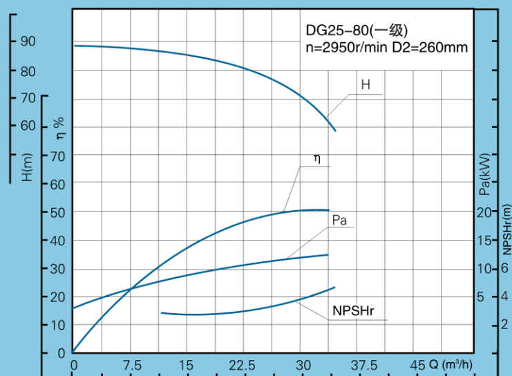
DG25-80次高压泵性能表
