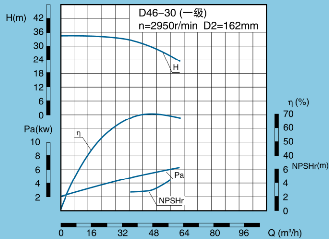
D、DG、DF、DY、DM46-30 性能表
