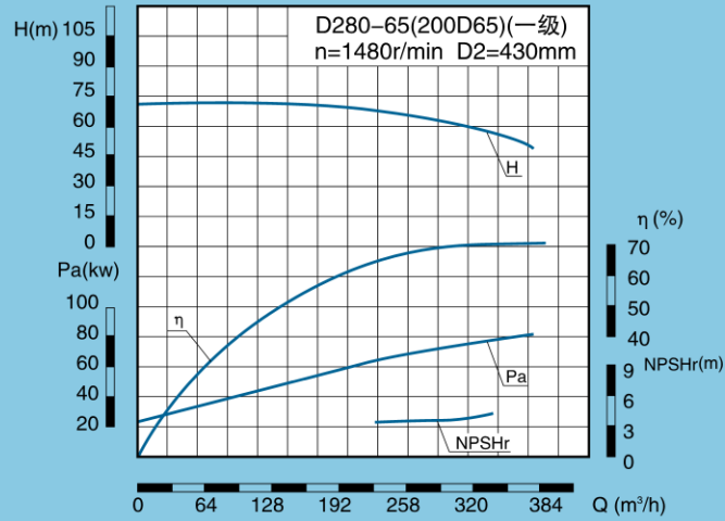
D、DG、DF、DY、DM280-65(200D65) 性能表
