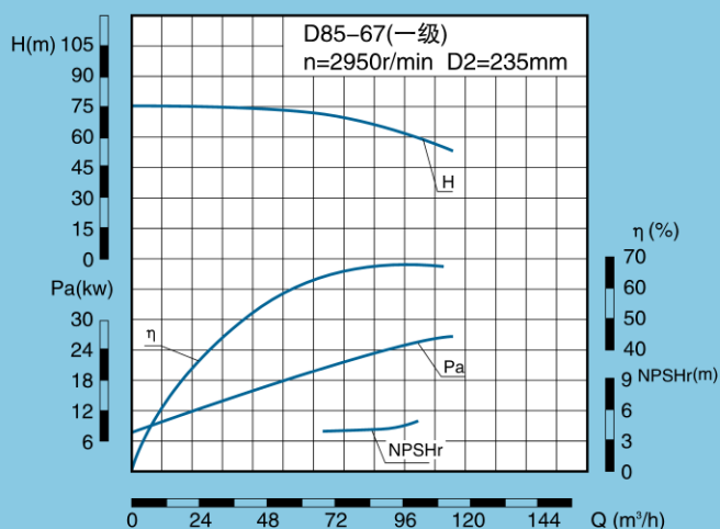
D、DG、DF、DY、DM85-67 性能表
