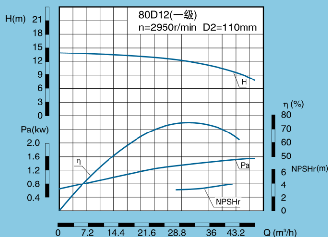
80D、DG、DF、DY、DM12 性能表
